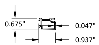
57 EXT. GLASS STOP-MONO. 6063-T5
