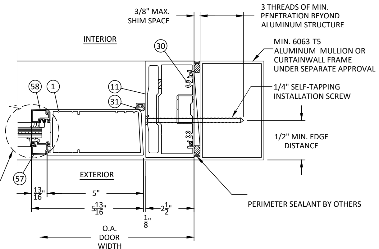
P HORIZONTAL SECTION 8 JAMB - ALUMINUM STUD
