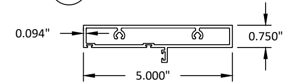
65 CW SUBFRAME - HEAD 6063-T5
