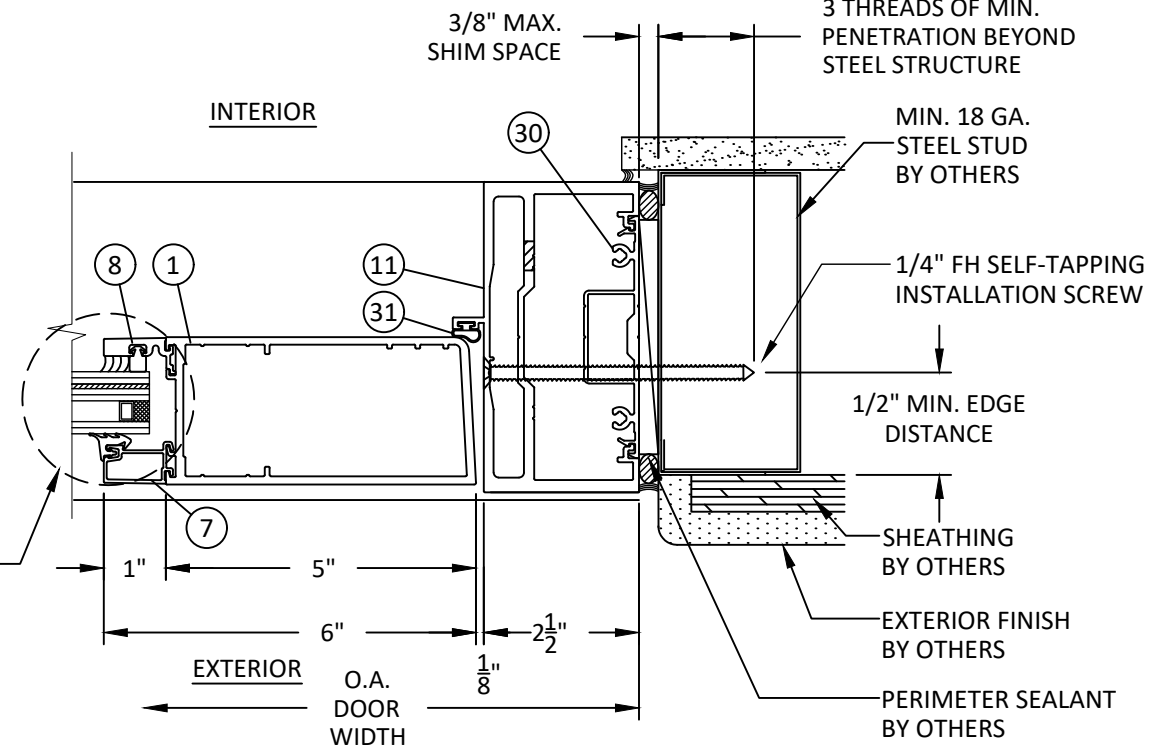
M HORIZONTAL SECTION 8 JAMB - STEEL STUD
