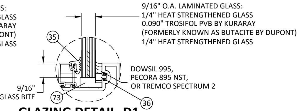
GLAZING DETAIL D1
