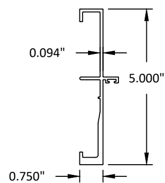
66 CW SUBFRAME - JAMBS 6063-T5
