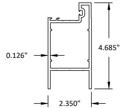
56 TOP RAIL - MONO. 6063-T5
